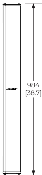
正面視圖
